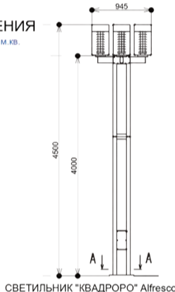
СВЕТИЛЬНИК "КВАДРО" Alfresco
