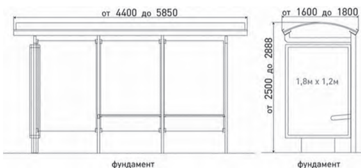
Чертежи внешнего вида
